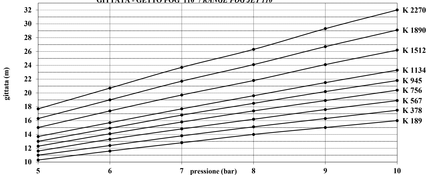
GITTATA - GETTO FOG 110° / RANGE FOG JET 110°
